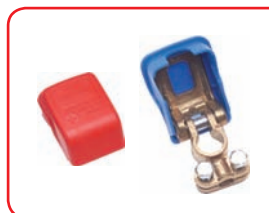
Sistema di chiusura a pressione Locking pressure system Ottone stagnato / Tin plated brass 1000 A - Cavo / Cable 16/50 mm 2 Cod. 40040
